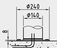
Gedübelt auf fertigen Fußboden (Standard)
