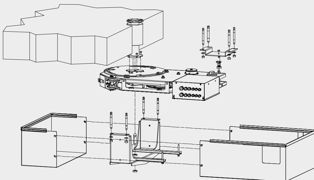
Antrieb unterflur
