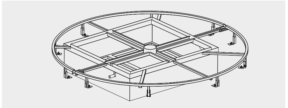
Bodenelement mit Antriebskasten für Bodengrube, ab Maß X = 350
